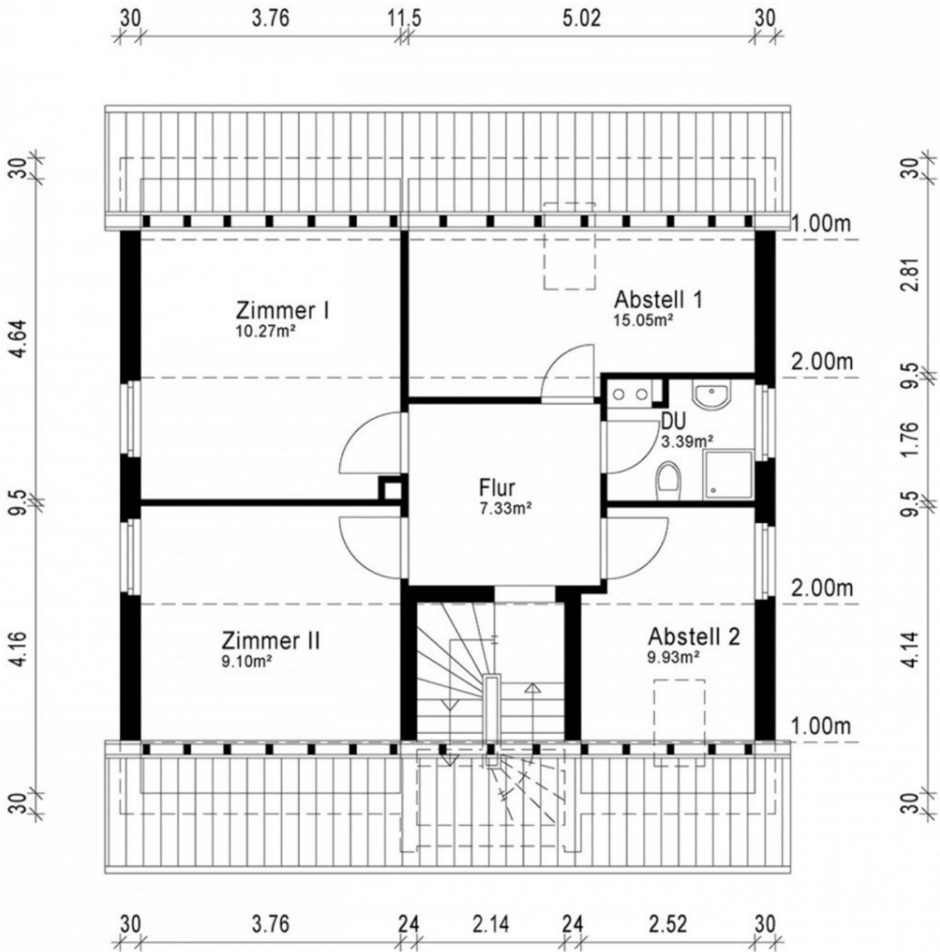
Grundriss DG
