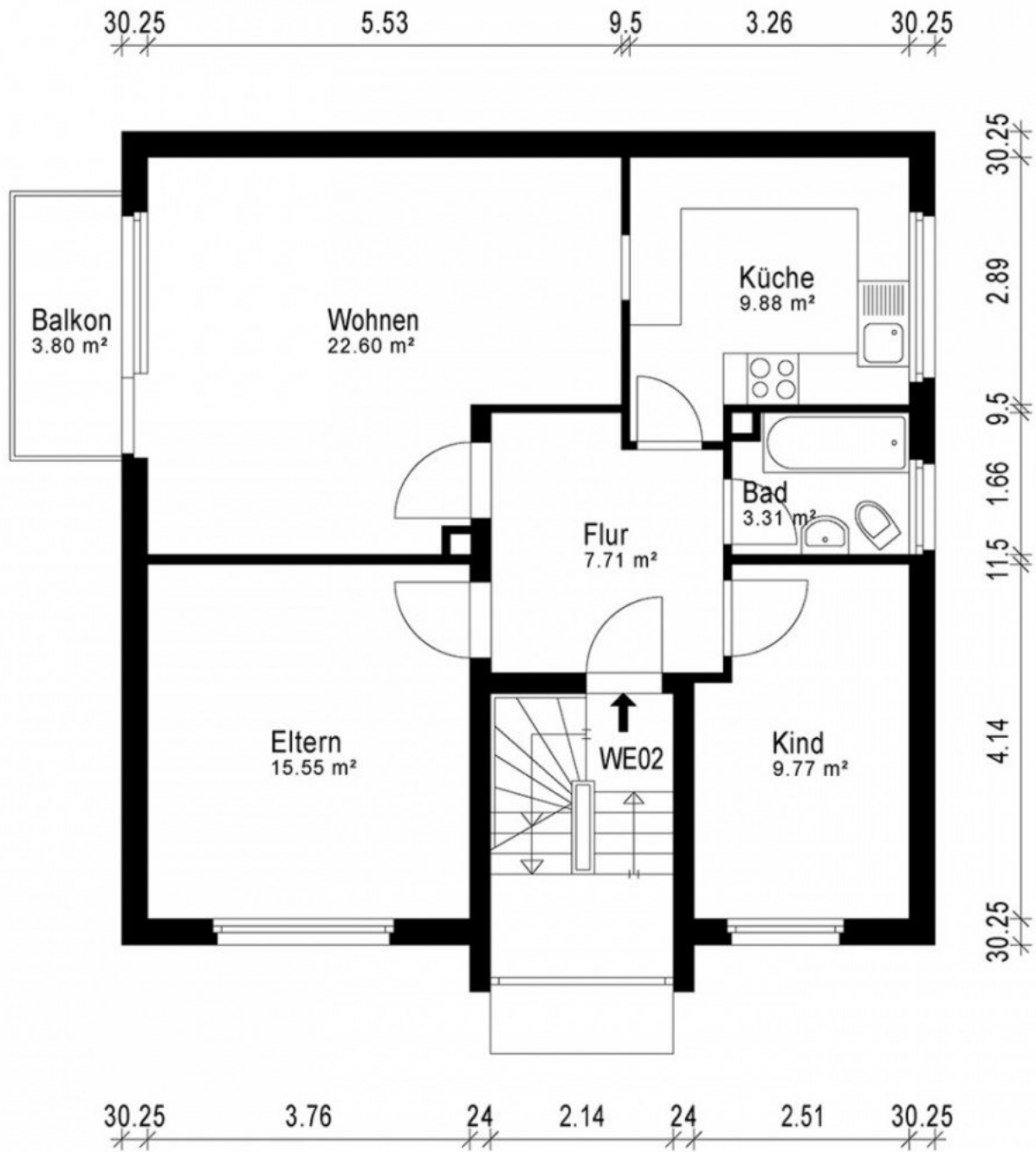
Grundriss OG
