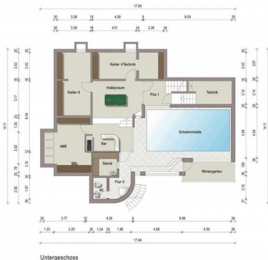
Untergeschoss
